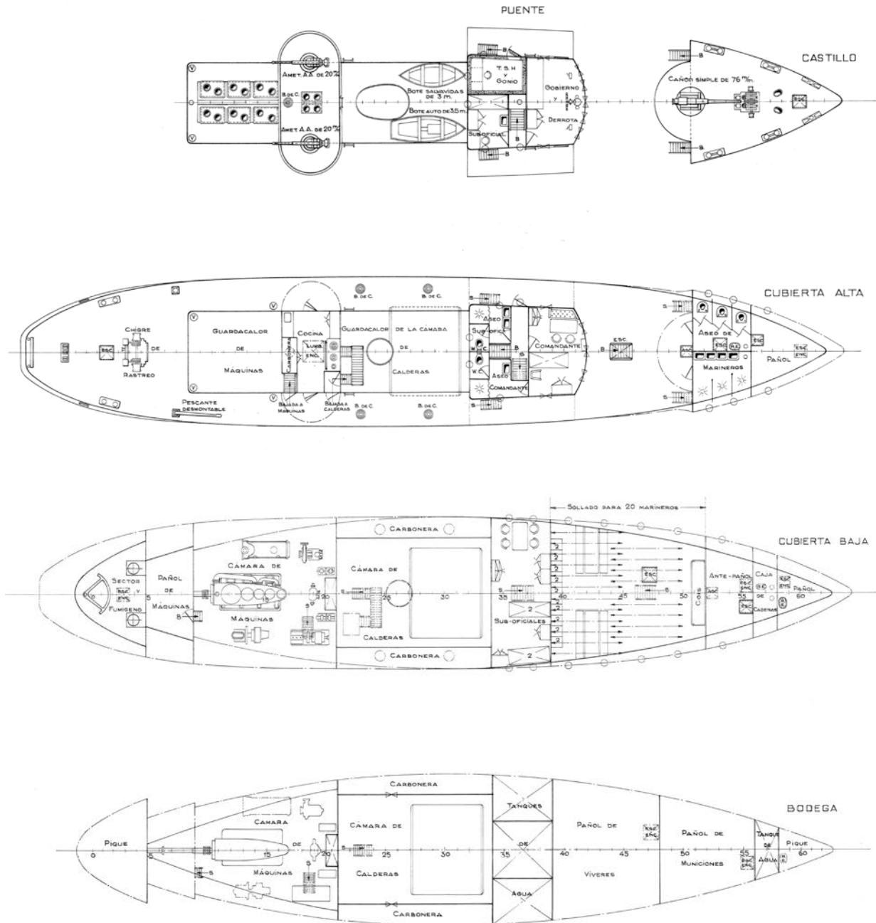
Рис. 47. Проект 42-R вид по палубам и надстройкам
