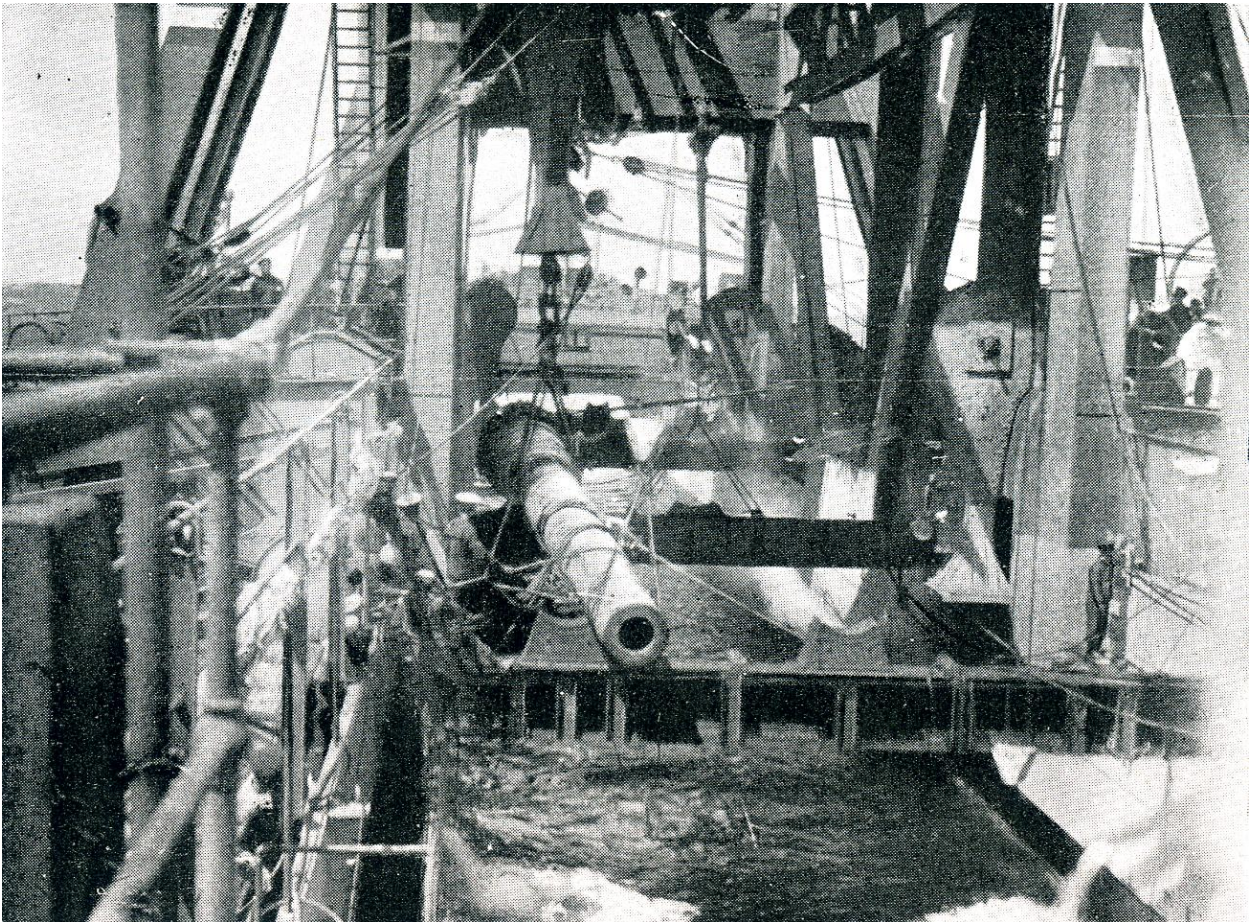
Рис. 29. Размещение одного из орудий на «Kanguro» ( Miranda y Maristany, 1924 )
