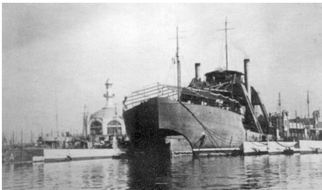
Рис. 40. «Kanguro» в сопровождении подводных лодок типа «В» ( Algo. 1 7 1933 № 203: 4 )
