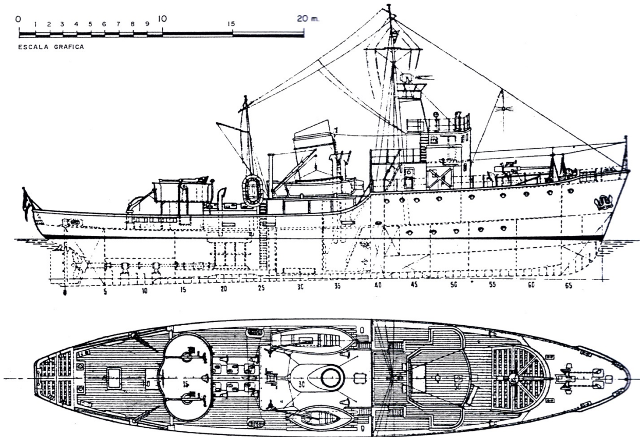
Рис. 50. Внешний вид судов береговой обороны (Coello Lillo, 2000)
